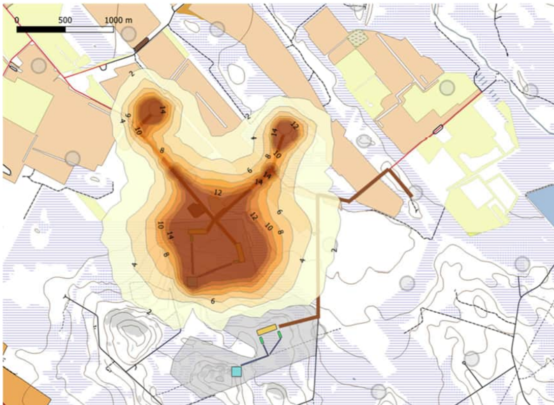
Kuva 13-7. Vaihtoehto VE2, PM10 pitoisuuden 50 \mu\text{g}/\text{m}^3 ylittävien päivien osuus vuoden päivistä (%).
