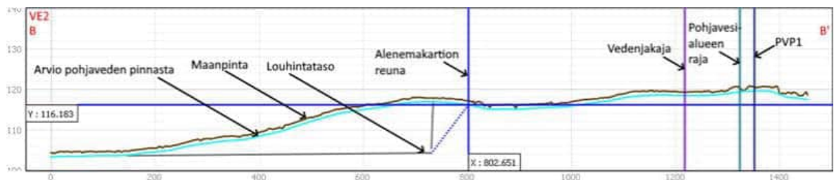
Kuva 11-8. Pituusleikkaus B-B' (Kuva 11-6) lävistäen ottoaluetta VE2. Leikkauksen kulku on karkeasti kohti Siikaniemenkallion huippua. Alenemakartio on suurin tässä kohtaa, yltyen noin 75 m louhosseinästä. Etäisyys pohjavesialueen rajaan on noin 500 m. Pohjavesialue on toisen pienvaluma-alueen puolella. Kuvassa on esitetty arvioitu pohjavesipinta havaintoputkien syvyyystiedon ja topografian perusteella (noin 1 m maanpinnasta).
