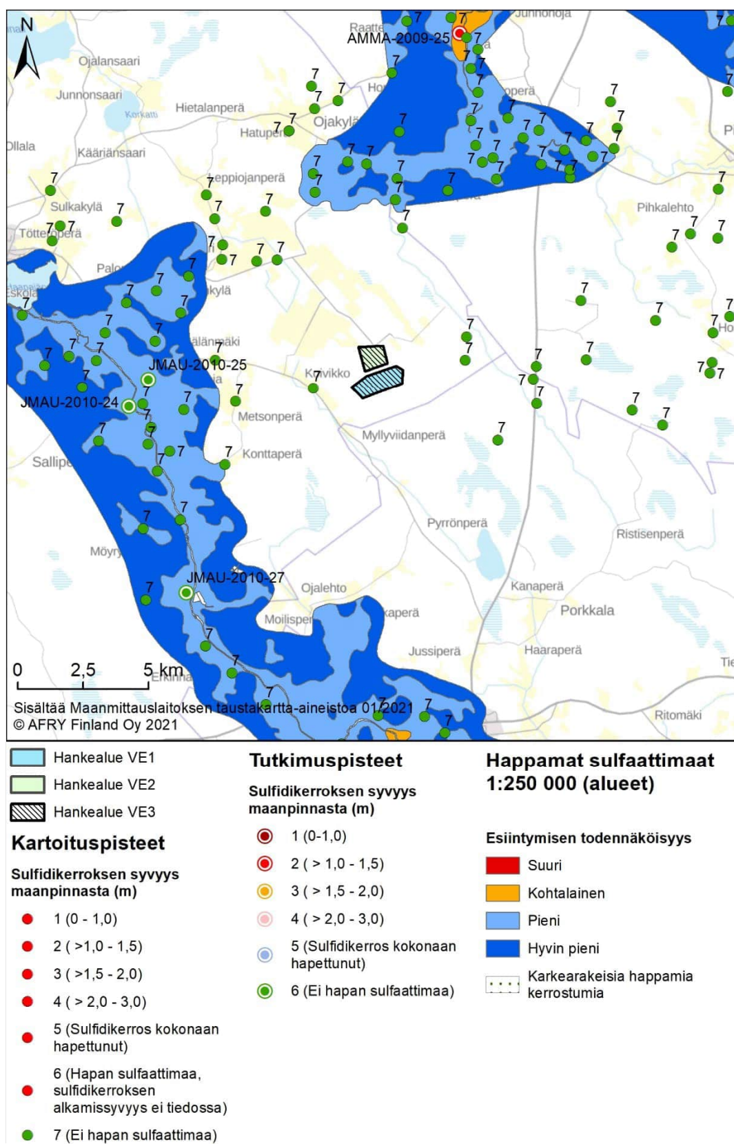
Kuva 11-3. Happamat sulfaattimaat (GTK 2021b).
