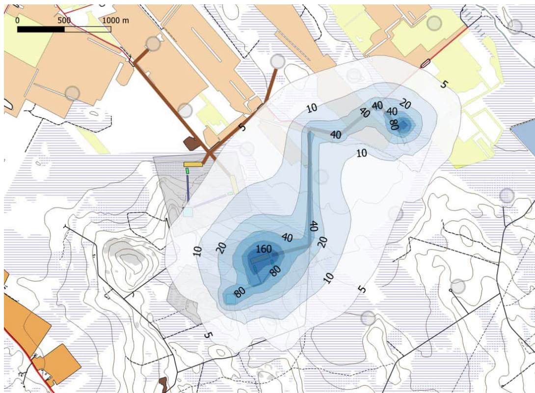
Kuva 13-2. Vaihtoehto VE1, PM10 vuoden keskipitoisuus \mu\text{g}/\text{m}^3 .
